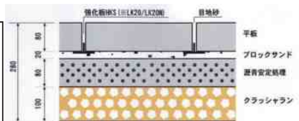
■ 格子パターンはH35、ブリックパターンはLK20/LK20Wを全T目地に挿入
