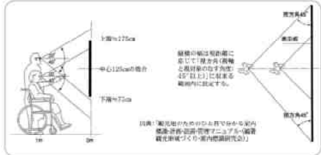
【歩行者系案内標識の見出し高さ・幅の考え方】
