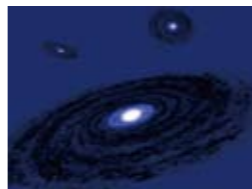
銀河はダークマターに囲まれているのだから
