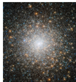
M15
