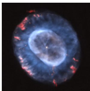
NGC 7662
