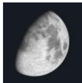
月(月齢10)
