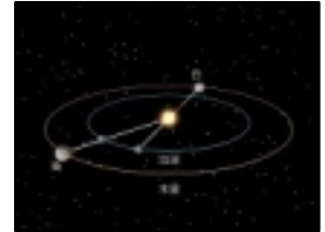
惑星の衝と合
