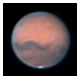
火星 (画像：国立天文台)
