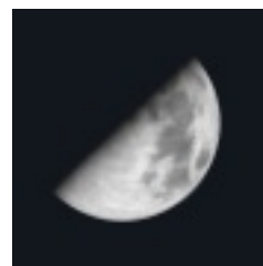
月（上弦）
