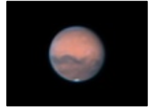
2020年の火星 画像：国立天文台
