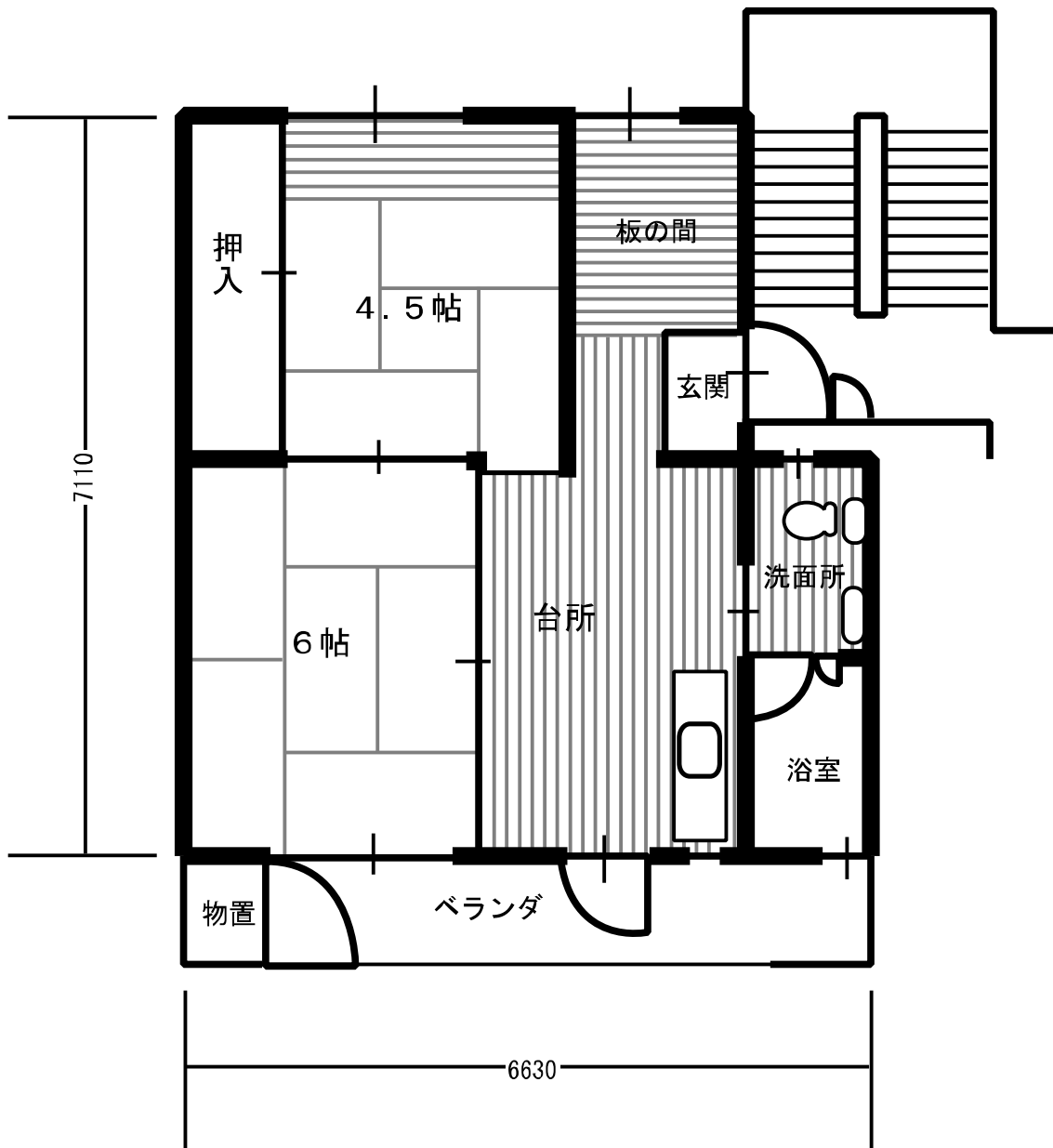
5・6号棟 (中層耐火・2UDK)
