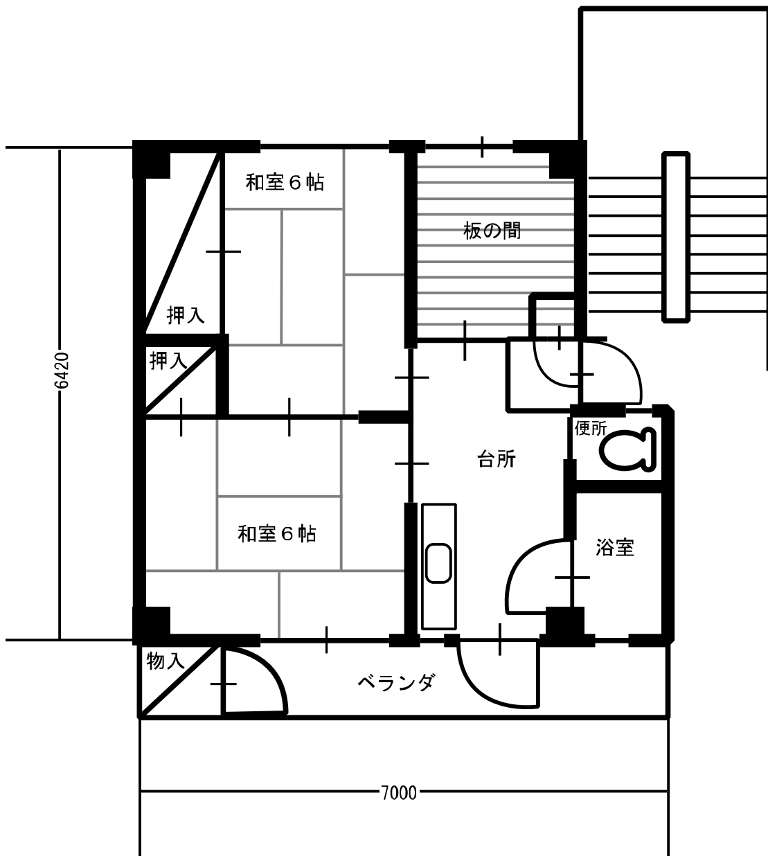
3号棟 (中層耐火・2UDK)
