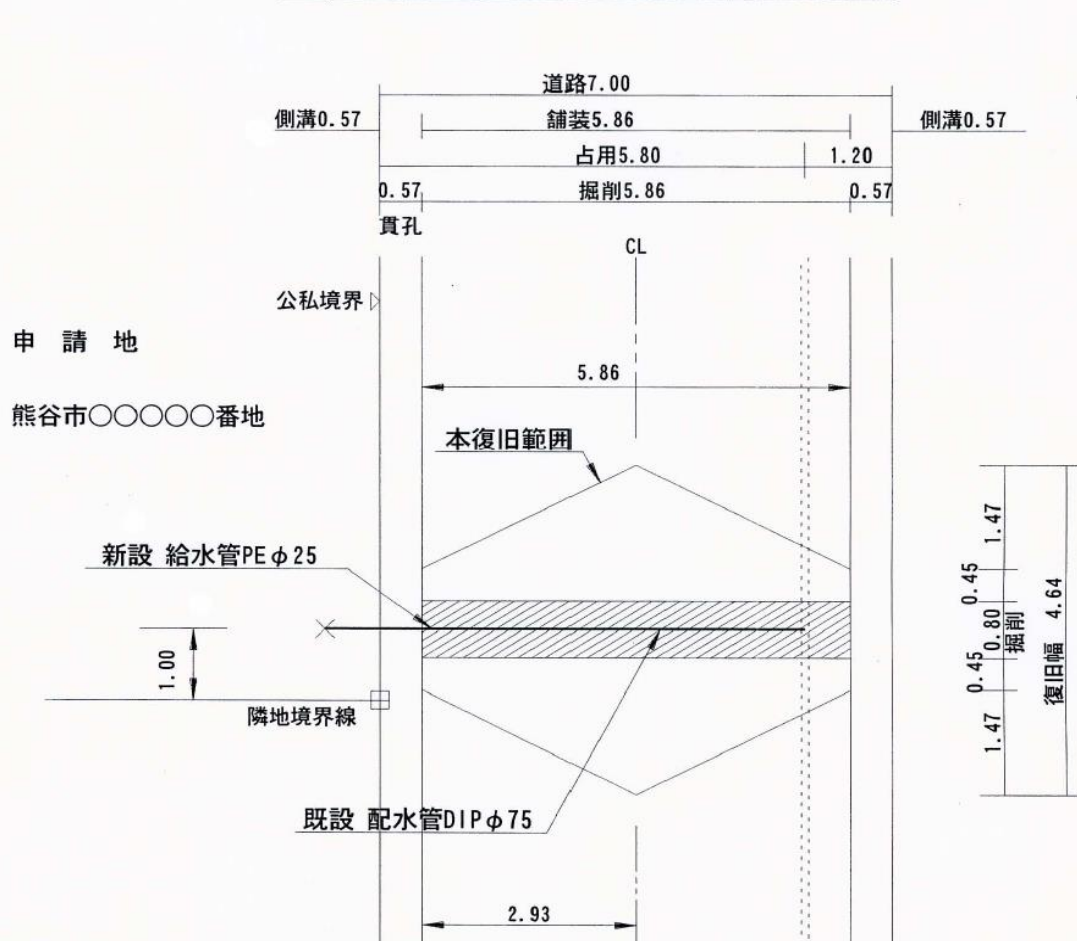
平面図 S=1/100 (単位：m)
