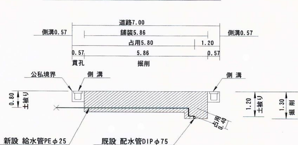
断面図 S=1/100 (単位：m)
