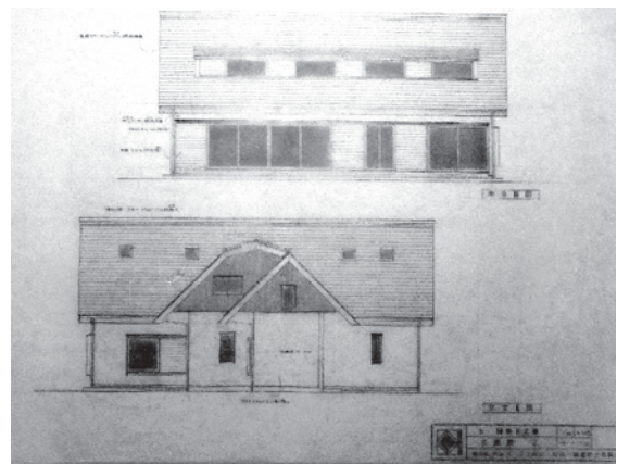
西村さんが描いた設計図
