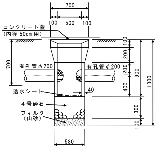
浸透枡構造図(標準)
