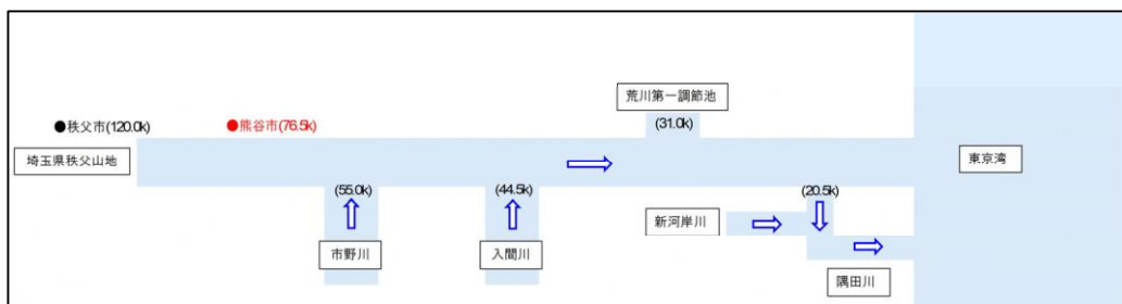
図2 荒川流域図
