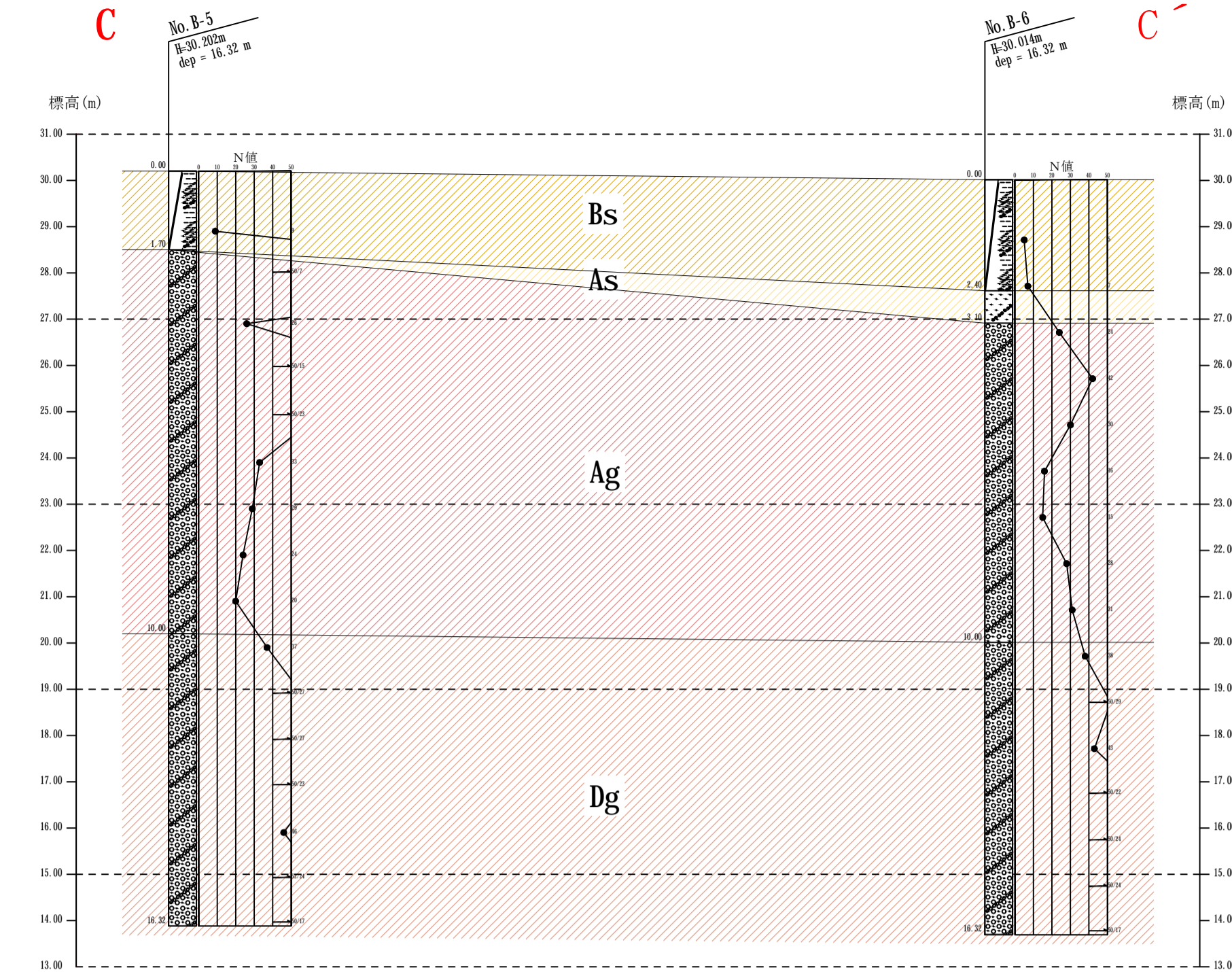
地層想定断面図 縮尺 H=1/1000 V=1/200
