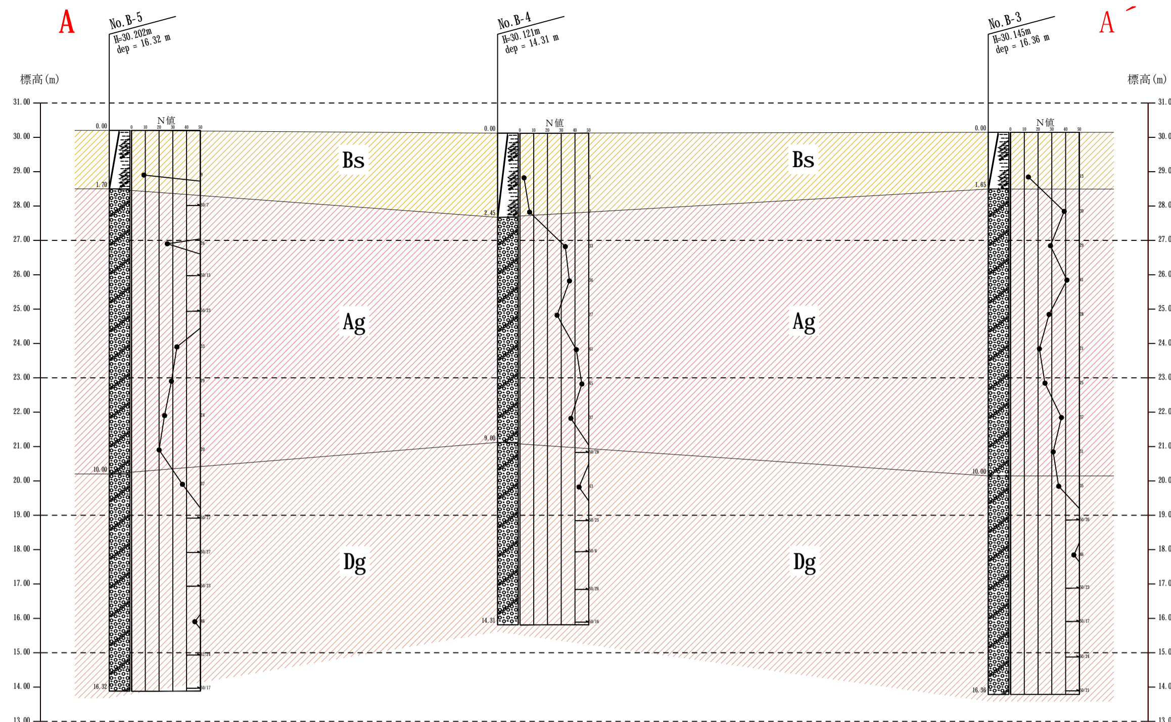
地層想定断面図 縮尺 H=1/1000 V=1/200
