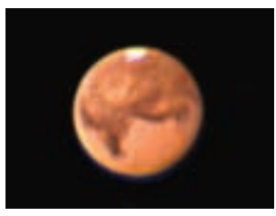
2003年夏の火星
