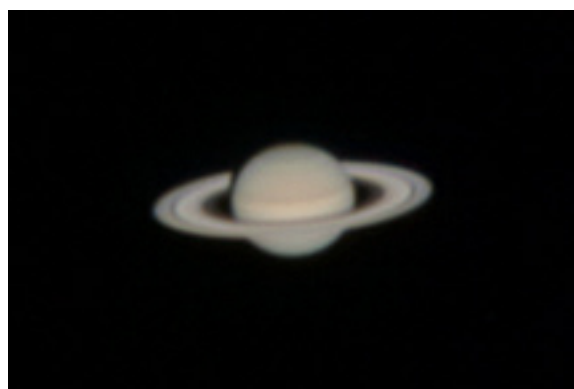
土星(画像：国立天文台) ※2022年撮影
