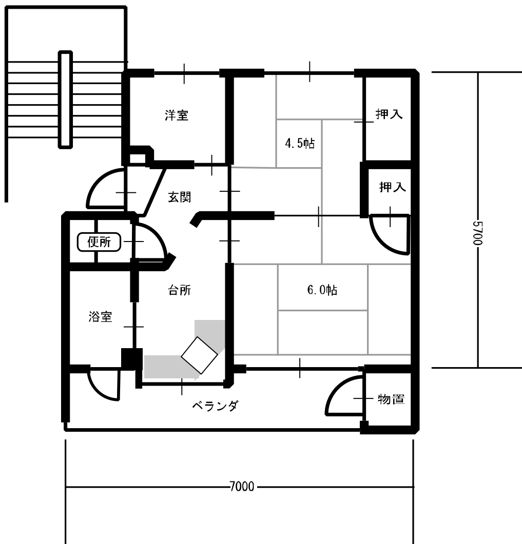
1号棟(中層耐火・2UDK)
