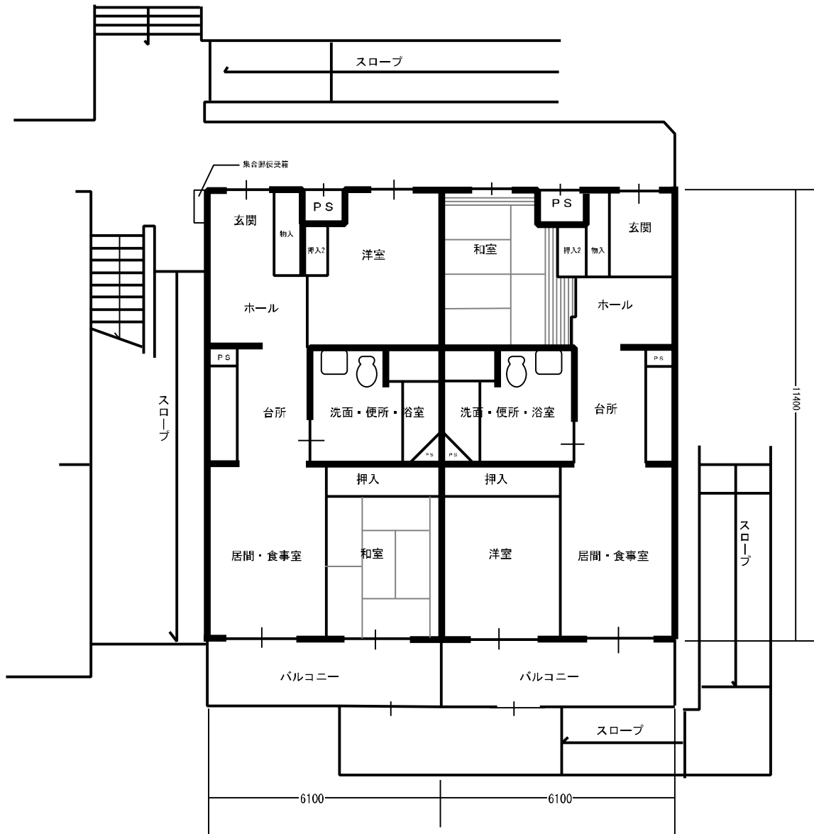
10号棟Nタイプ[2戸] (中層耐火・2LDK・車椅子用)
